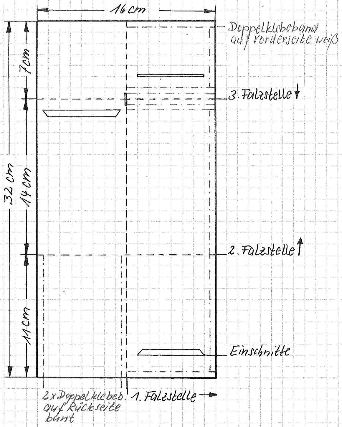
Vorlagenskizze Maßstab 1:2
